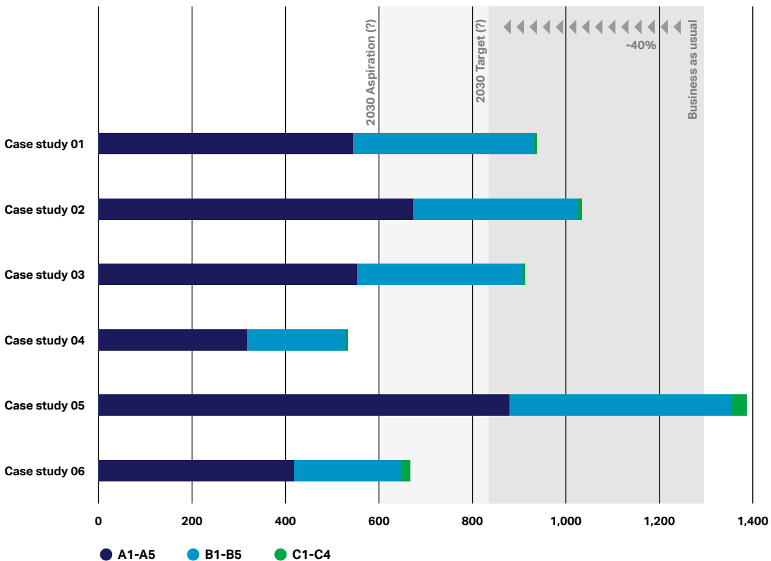
Figure 37: A-C per case study (kgCO2e/m²)
